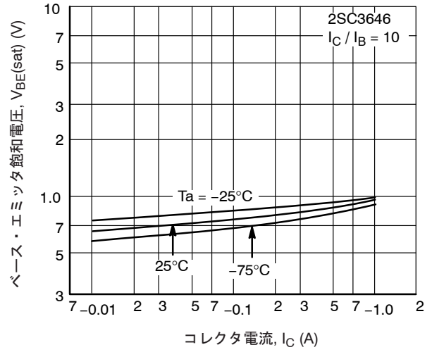
図 14. V_{BE(sat)} - I_C
