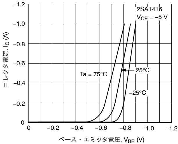
図 5. I_C - V_{BE}
