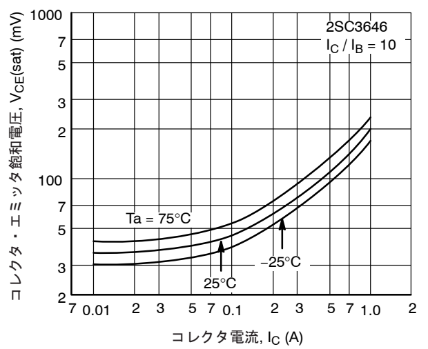
図 12. V_{CE(sat)} - I_C
