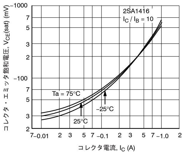
図 11. V_{CE(sat)} - I_C
