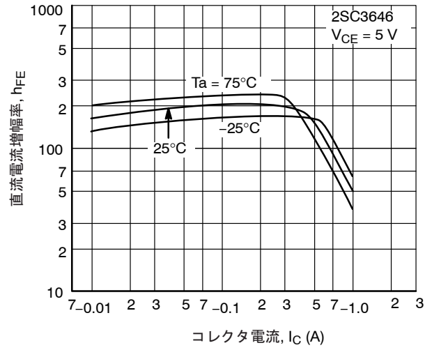
図 8. h_{FE} - I_C
