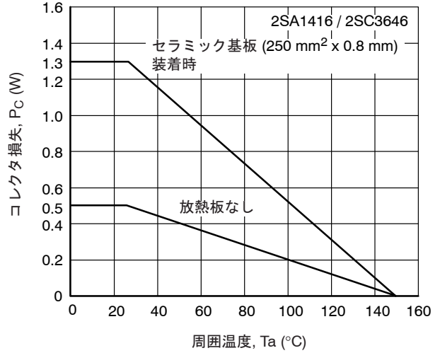
図 16. P_C - T_a
