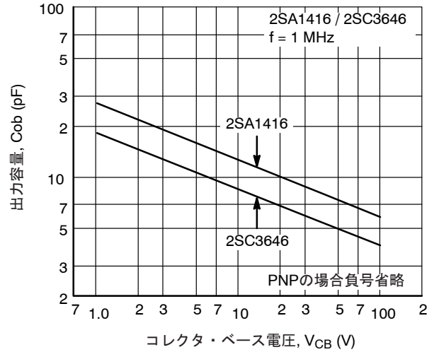
図 10. C_{ob} - V_{CB}
