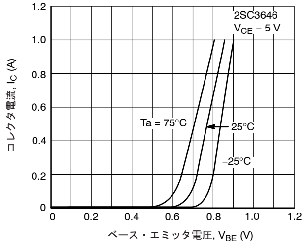
図 6. I_C - V_{BE}
