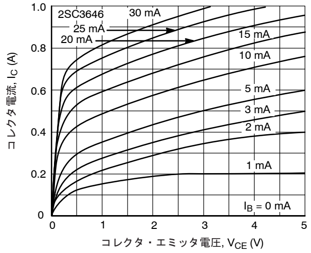
図 2. I_C - V_{CE}
