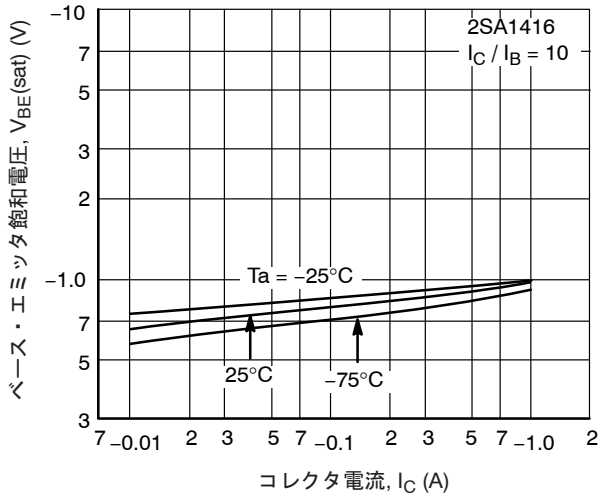
図 13. V_{BE(sat)} - I_C
