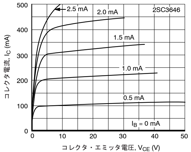
図 4. I_C - V_{CE}
