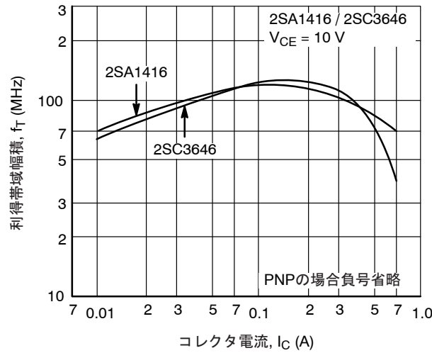
図 9. f_T - I_C
