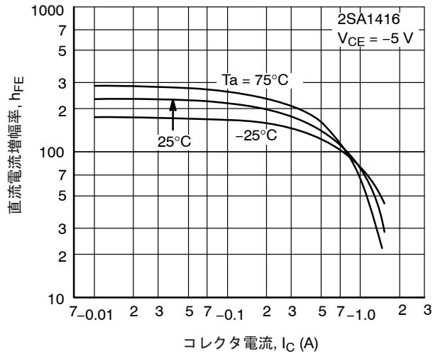
図 7. h_{FE} - I_C
