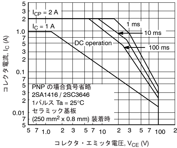
図 15. ASO
