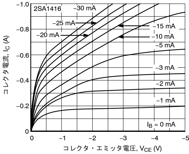
図 1. I_C - V_{CE}
