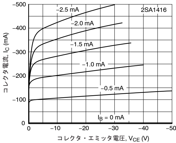
図 3. I_C - V_{CE}
