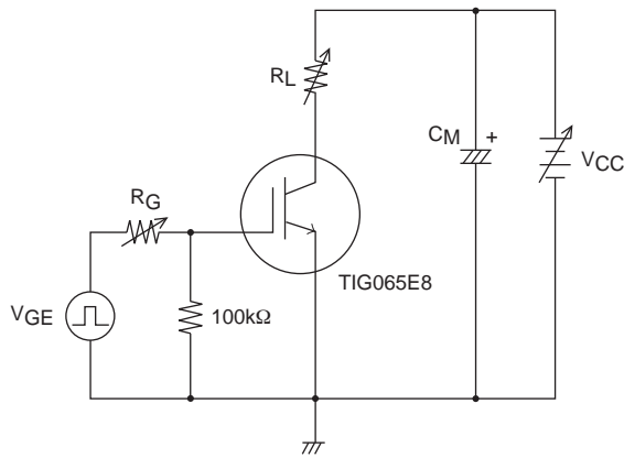
図1 大電流 R 負荷スイッチング回路図
