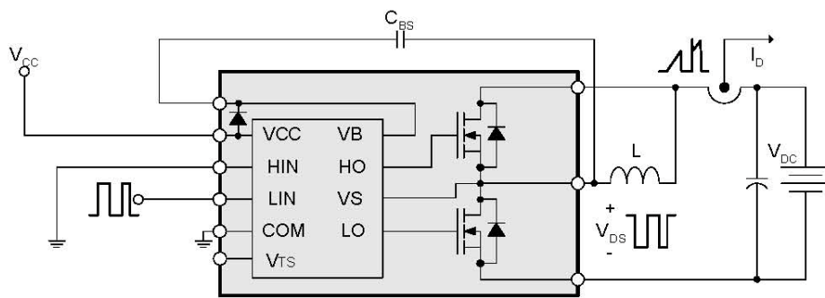
Motion SPM ® 5 製品 1 相分のブロック図
