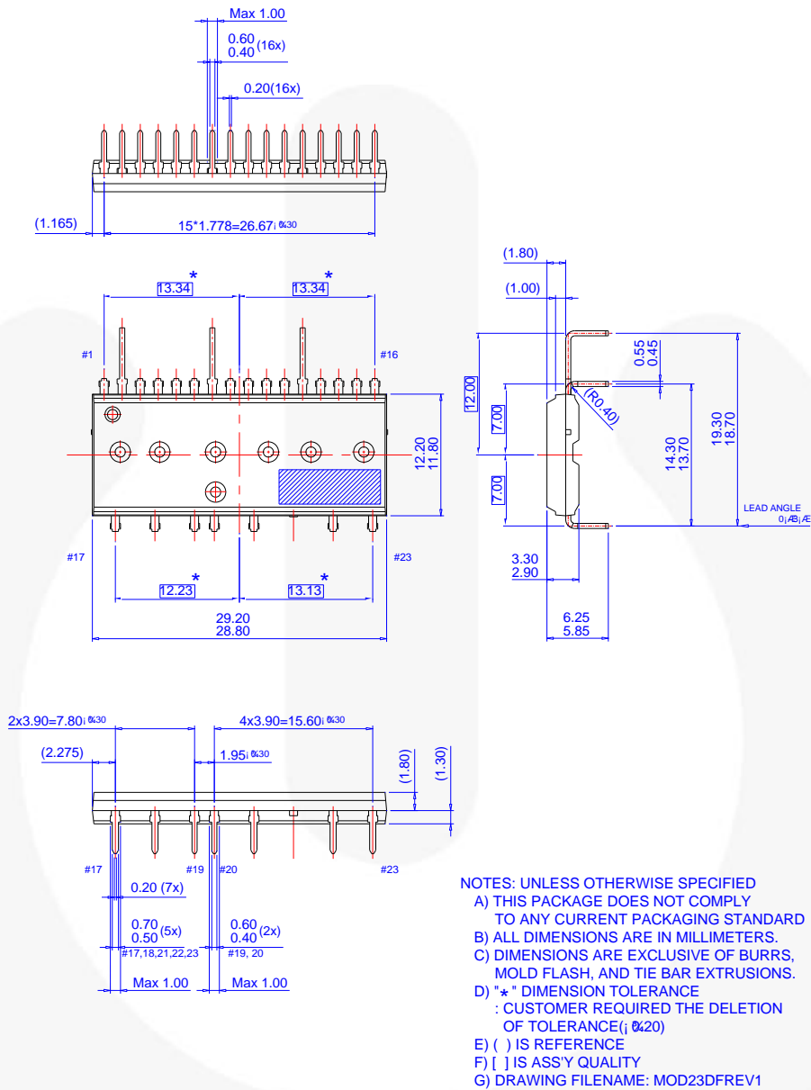
图 12. 寸法単位 : [mm]
