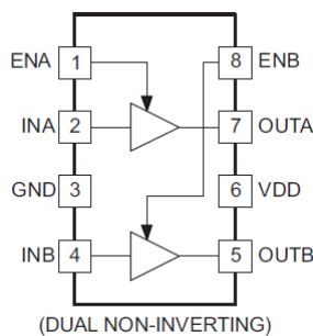
NCP81071B
