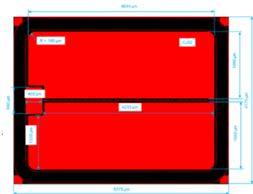
DIE OUTLINE
