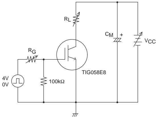
図1 大電流 R 負荷スクリーニング回路図
