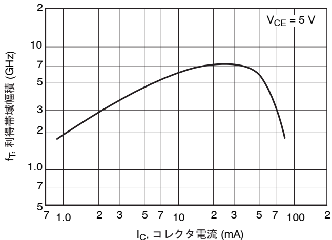
図 2. f_T - I_C
