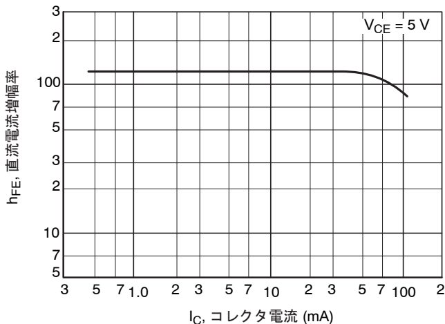
図 1. h_{FE} - I_C
