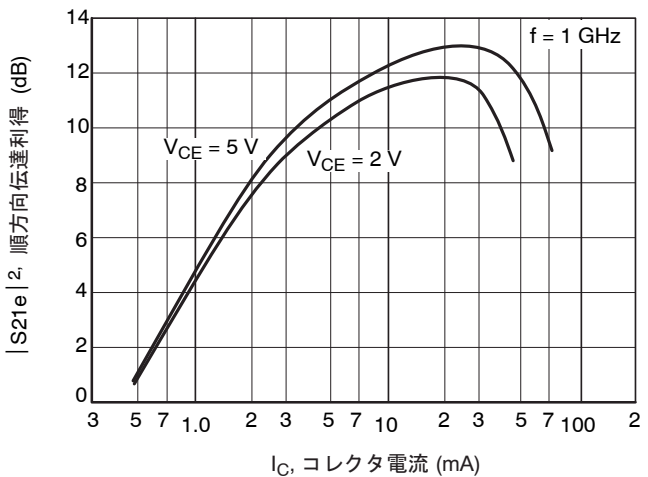
図 6. |S_{21e}|^2 - I_C
