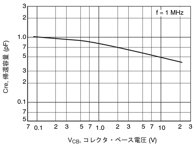
図 4. C_{re} - V_{CB}
