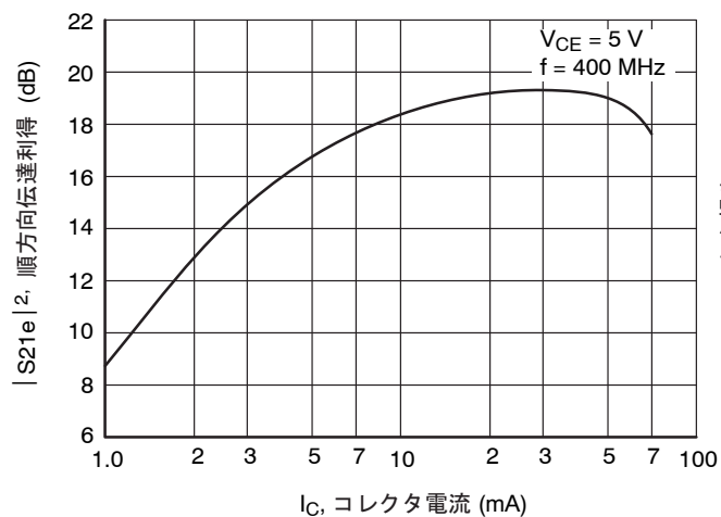
図 9. |S_{21e}|^2 - I_C
