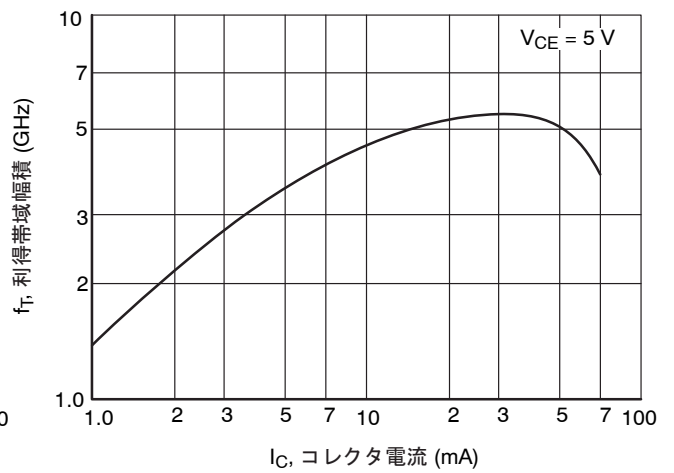
図 4. f_T - I_C
