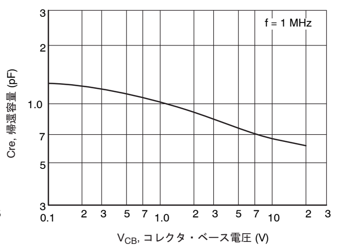
図 6. C_{re} - V_{CB}
