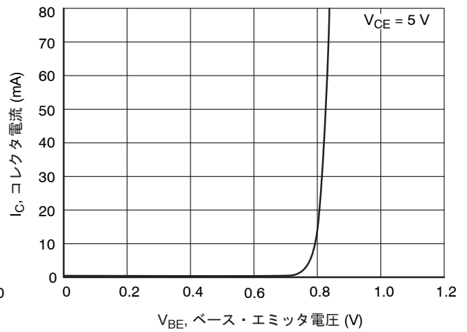
図 2. I_C - V_{BE}
