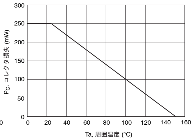
図 10. P_C - T_a
