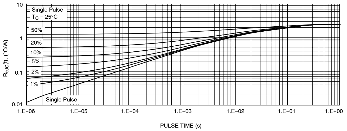
图 14. Thermal Response
