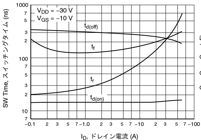
図 8. SW Time - I_D
