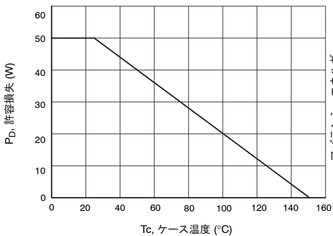
図 12. P_D - T_C
