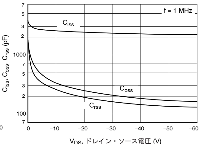
図 9. C_{iss} , C_{oss} , C_{rss} - V_{DS}
