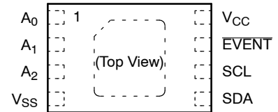
TDFN (VP2)
