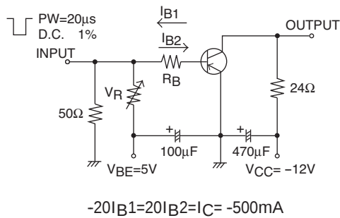
スイッチングタイム測定回路図
