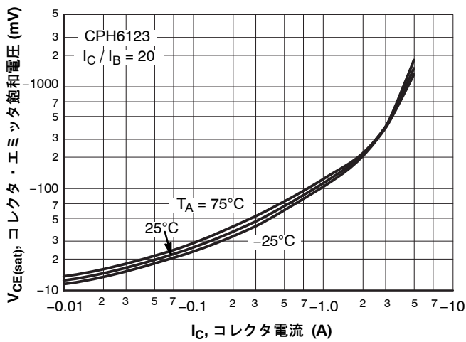
図 12. V_{CE(sat)} - I_C
