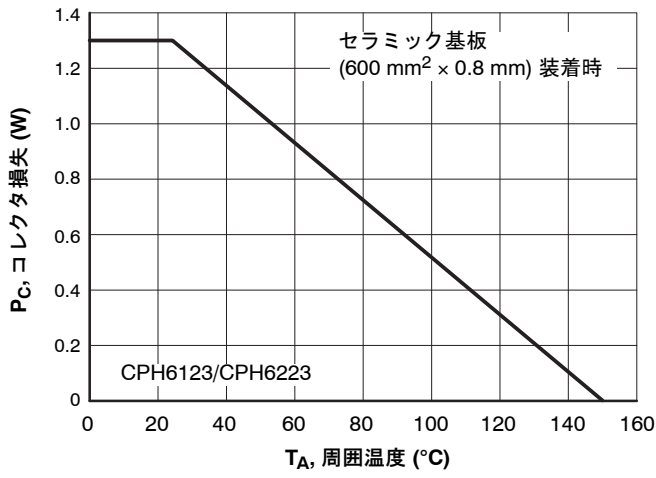
図 20. P_C - T_A
