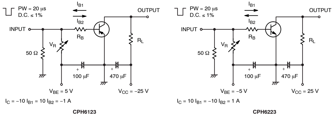
図 1. スイッチングタイム測定回路図
