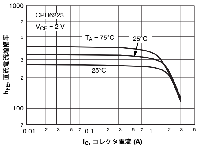
図 7. h_{FE} - I_C
