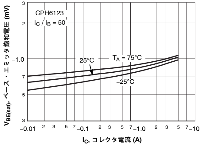
図 16. V_{BE(sat)} - I_C
