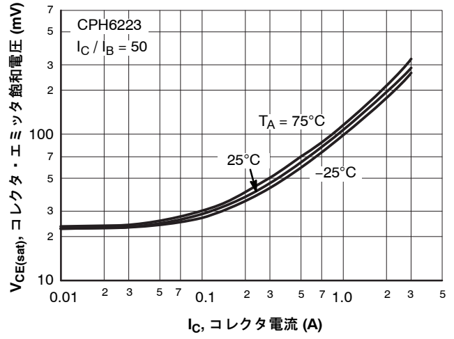
図 15. V_{CE(sat)} - I_C
