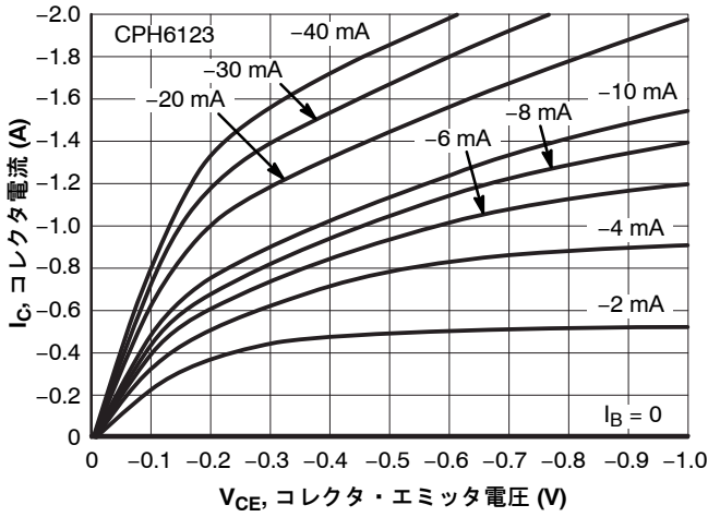
図 2. I_C - V_{CE}
