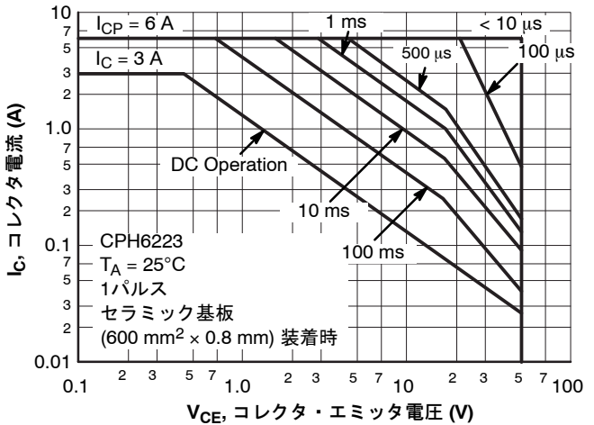
図 19. ASO
