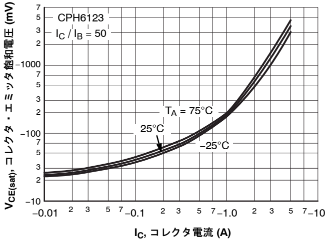
図 14. V_{CE(sat)} - I_C
