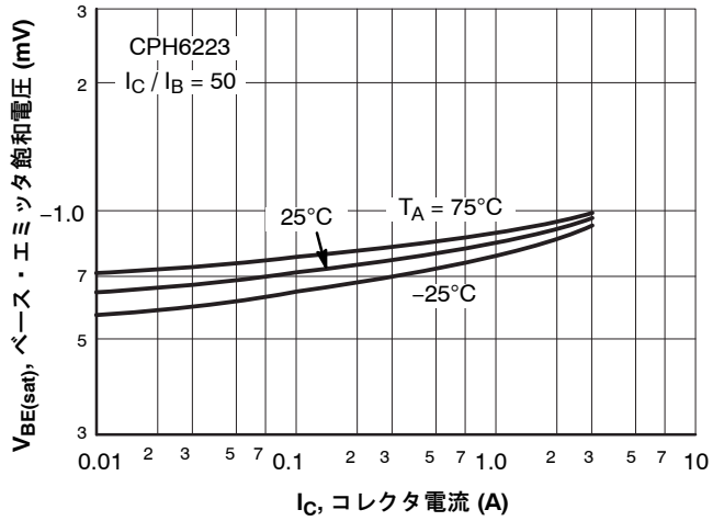
図 17. V_{BE(sat)} - I_C
