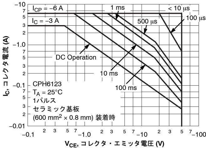
図 18. ASO
