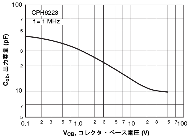
図 11. C_{ob} - V_{CB}
