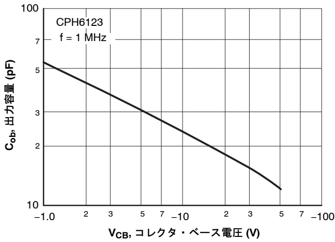
図 10. C_{ob} - V_{CB}
