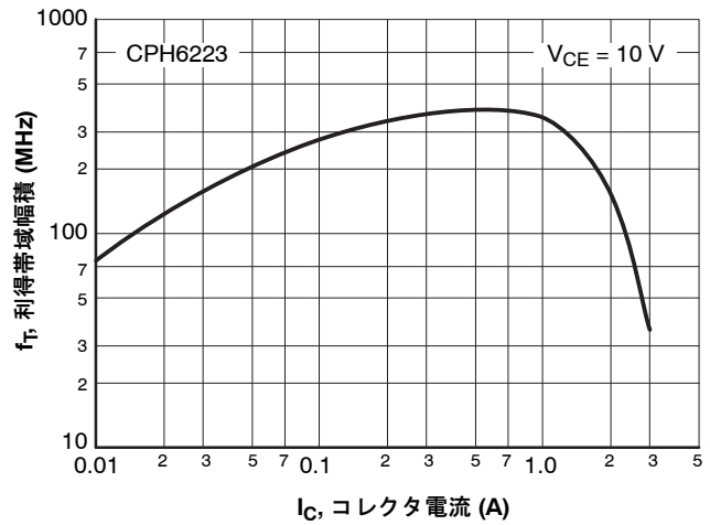
図 9. f_T - I_C
