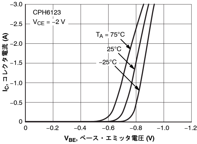
図 4. I_C - V_{BE}
