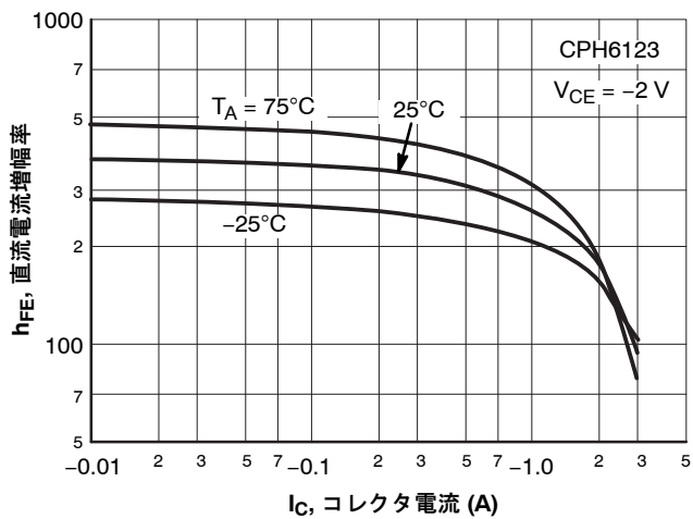
図 6. h_{FE} - I_C
