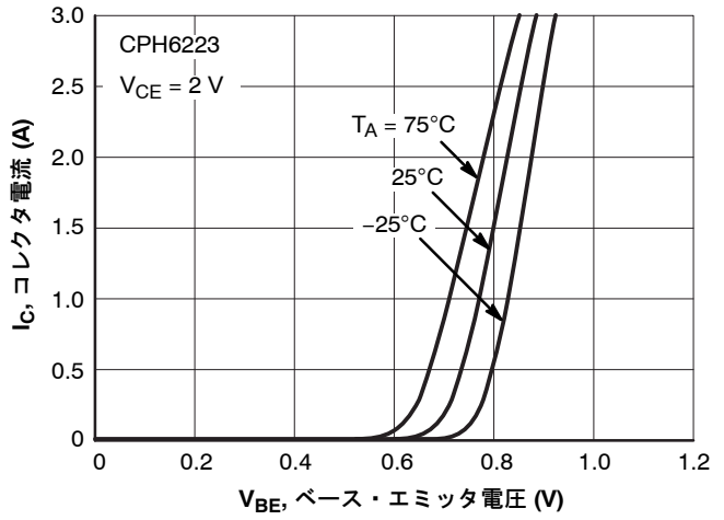
図 5. I_C - V_{BE}
