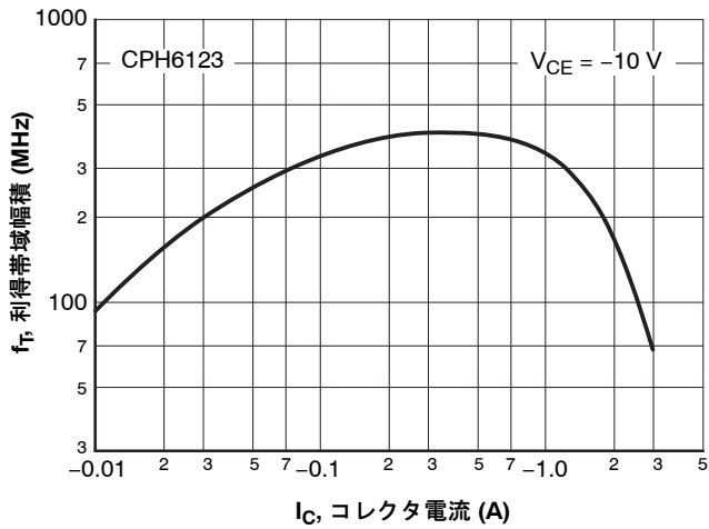
図 8. f_T - I_C
