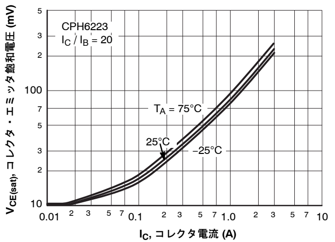
図 13. V_{CE(sat)} - I_C
