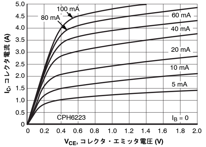
図 3. I_C - V_{CE}
