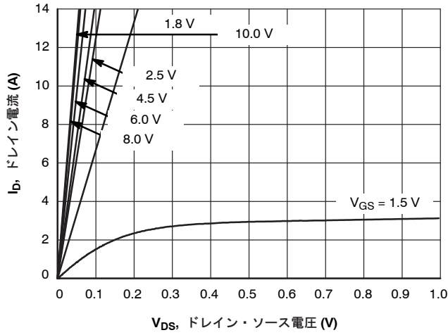
図 3. I_D - V_{DS}
