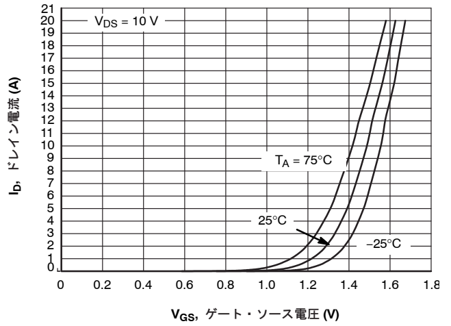
図 4. I_D - V_{GS}
