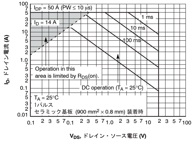
図 12. ASO
