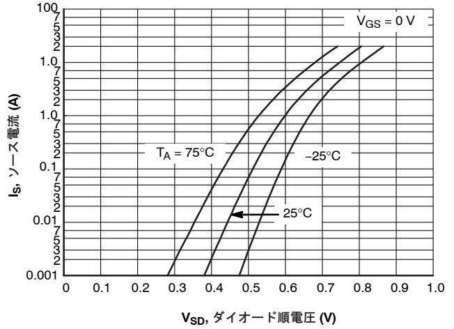
図 8. I_S - V_{SD}
