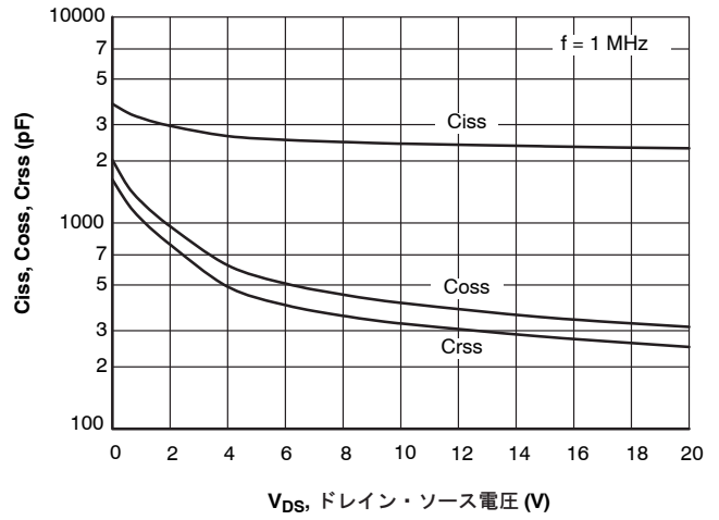
図 10. Ciss, Coss, Crss - V_{DS}
