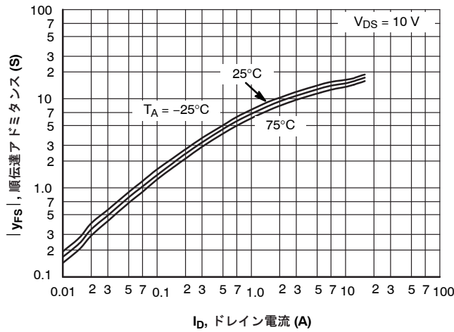
図 7. |y_{fs}| - I_D
