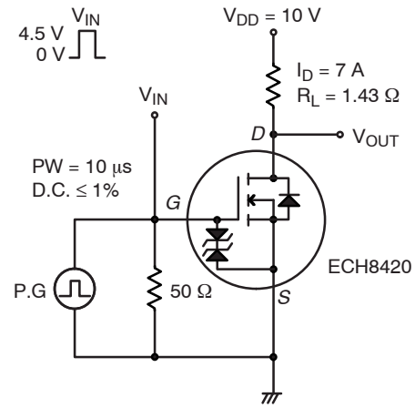
図 2. スwitchingタイム測定回路図
