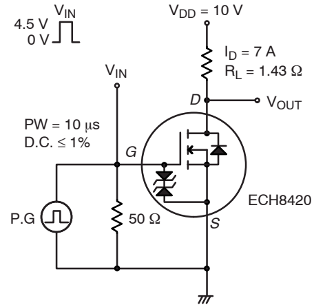
図 2. スwitchingタイム測定回路図
