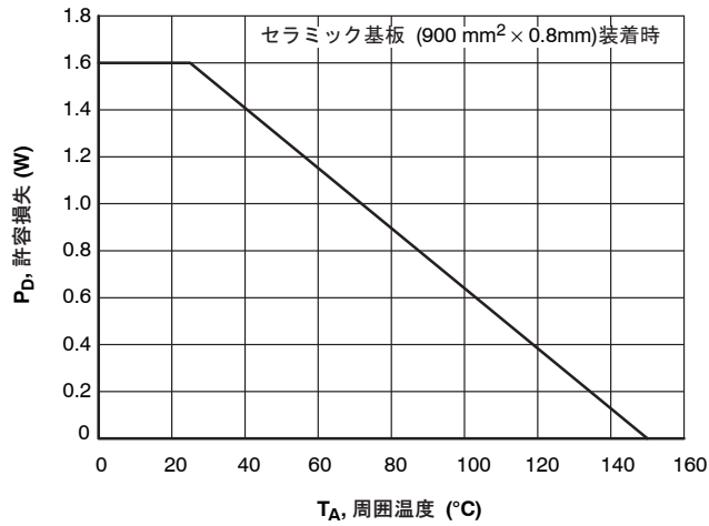
図 13. P_D - T_A
