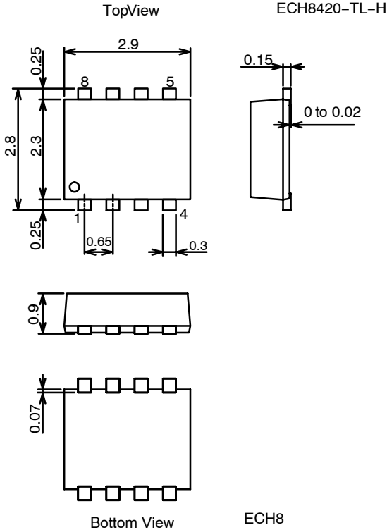
図 1. 外形図
