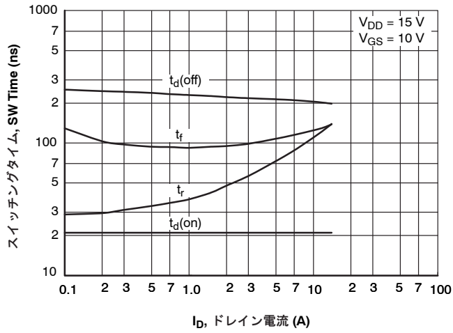
図 9. SW Time - I_D
