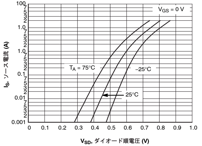
図 8. I_S - V_{SD}
