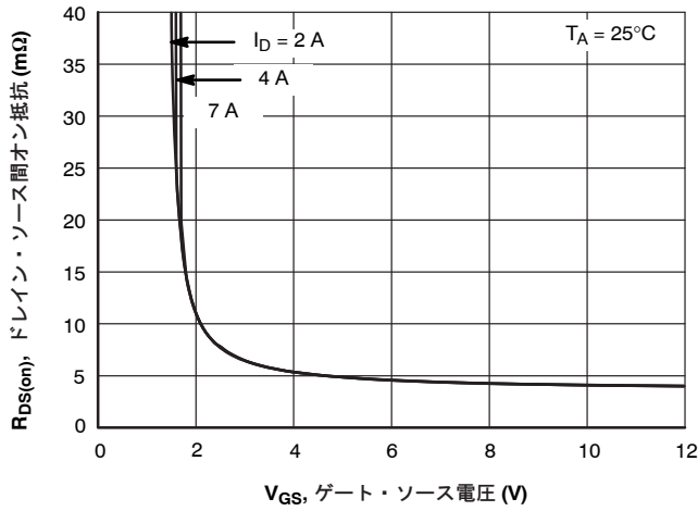
図 5. R_{DS(on)} - V_{GS}
