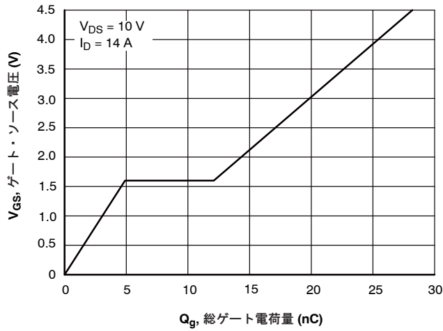
図 11. V_{GS} - Q_g
