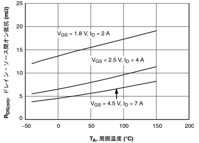
図 6. R_{DS(on)} - T_A
