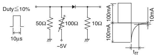
t rr 指定回路図
