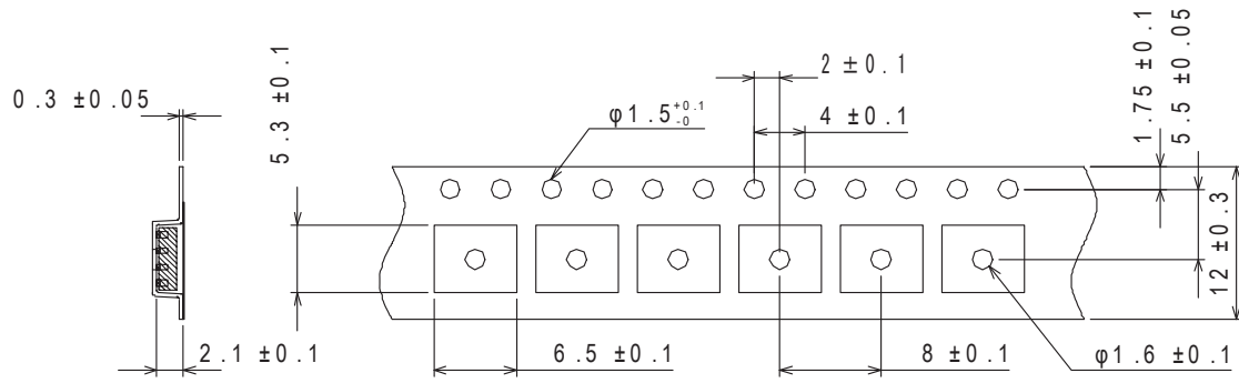
2-1. キャリアテープ寸法 (単位: mm)
