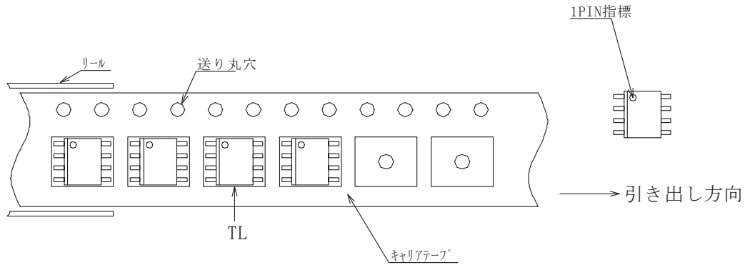
2-2. 部品の方向
