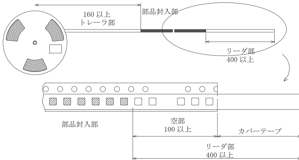
2-3. リーダ部及びトレーラ部 (単位: mm)
