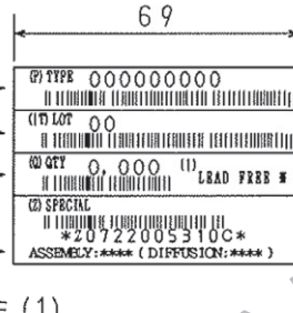
リールラベル, 内装箱ラベル (単位: mm)
