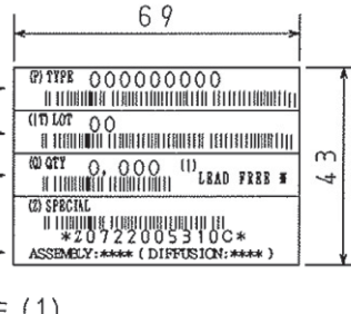
リールラベル, 内装箱ラベル (単位: mm)
