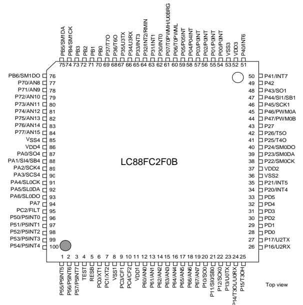
ピン配置図 (Top view)
