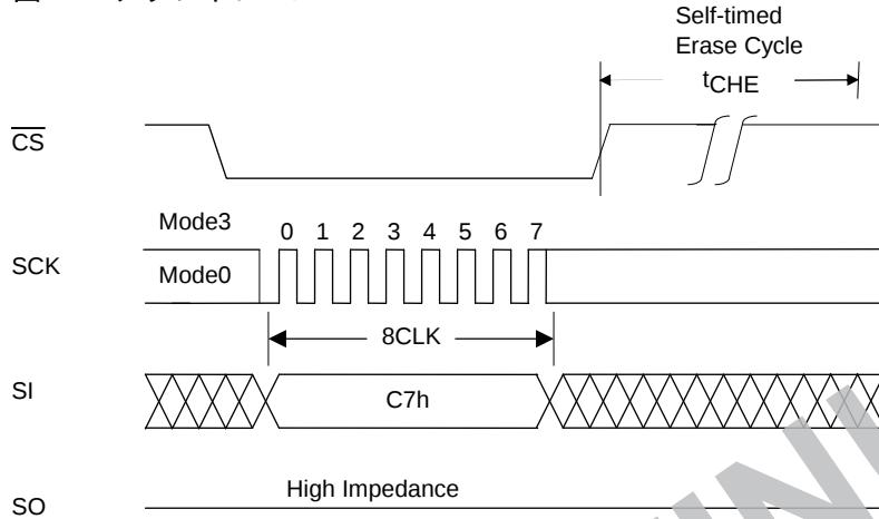
図 14：チップイレース
