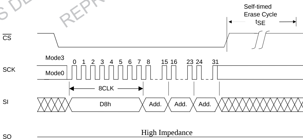
図 13：セクタイレース
