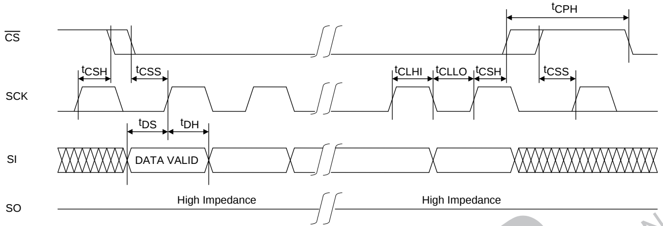
図 3 : シリアル入力タイミング
