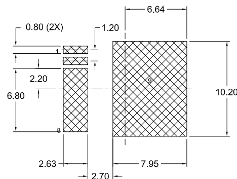
SECTION "A-A" SCALE: 2X
