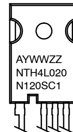
TO-247-4LD CASE 340CJ
