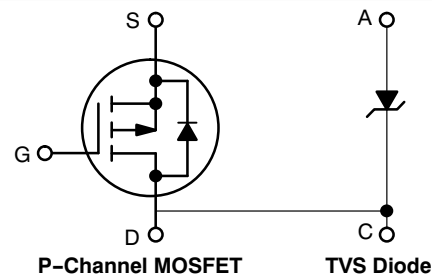
ChipFET CASE 1206A STYLE 6
