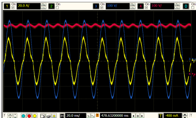
Figure 24. Vin 220 V, Pin = 4.95 kW
