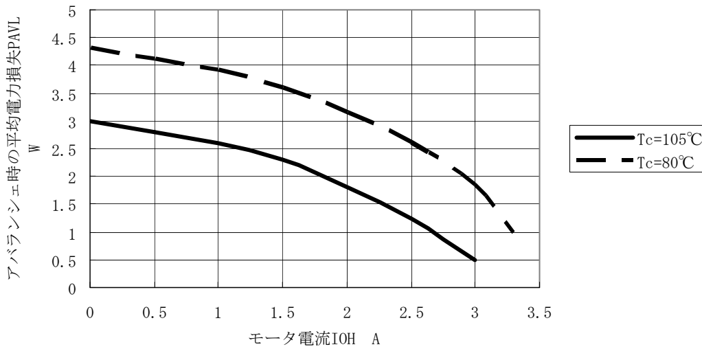
図-3 STK672-440BN-E アバランシェ動作時の許容損失範囲 PAVL-IOH
