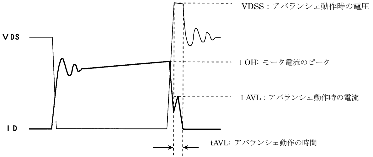
図-1 2 相ステッパモータを定電流チョッピング駆動させた時の STK672-4**シリーズの出力電流 ID,電圧 VDS 波形 1
