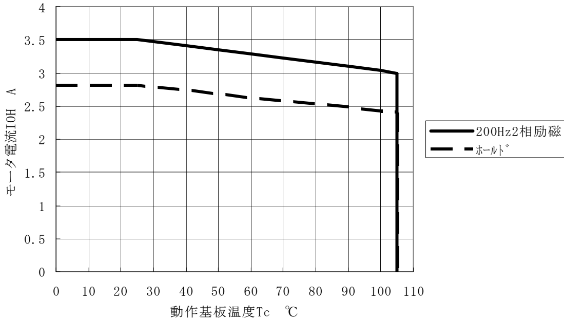
STK672-440BN-E 動作基板温度 T_c に対するモータ電流 I_{OH} の軽減曲線
