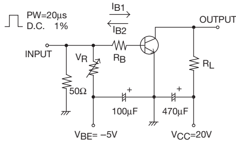
スイッチングタイム測定回路図
